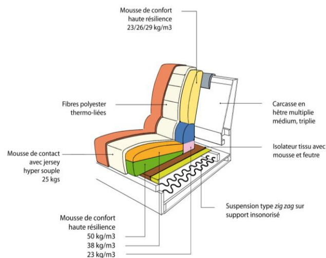
Détail pour le petit fauteuil
