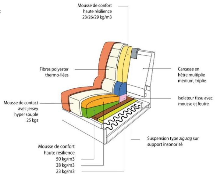
COUPE POUR LE PETIT FAUTEUIL
